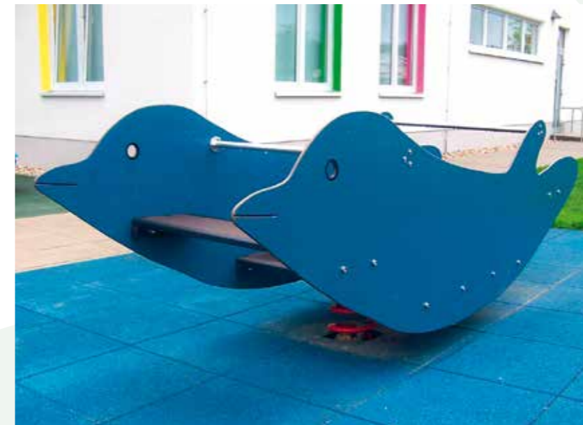
Mehrfachfederwippe „Delphin“
